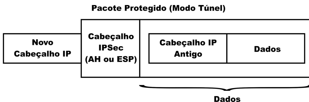
Figura 26: Modo túnel.
