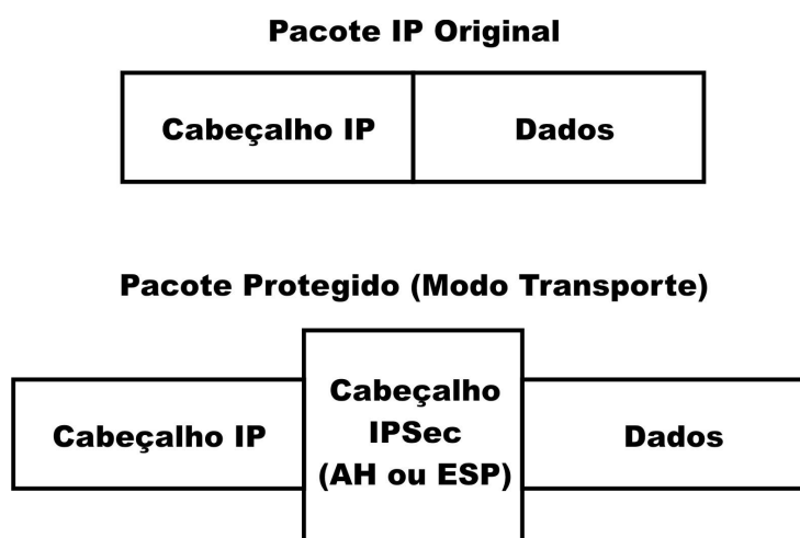
Figura 25: Modo transporte.
