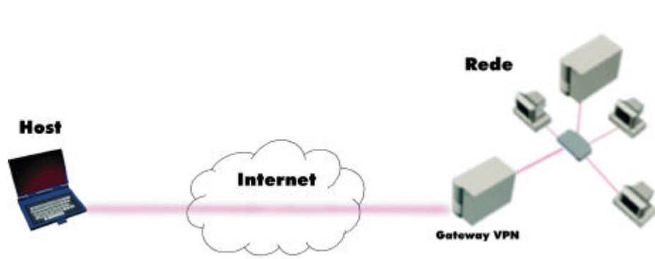
Figura 23: Topologia host-rede .
