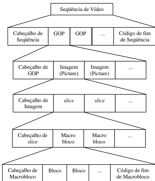
Figura 3: Estrutura da Camada de Vídeo MPEG
