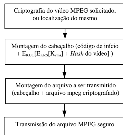
Figura 8: Fluxograma da Criptografia e Transmissão do Vídeo Seguro
