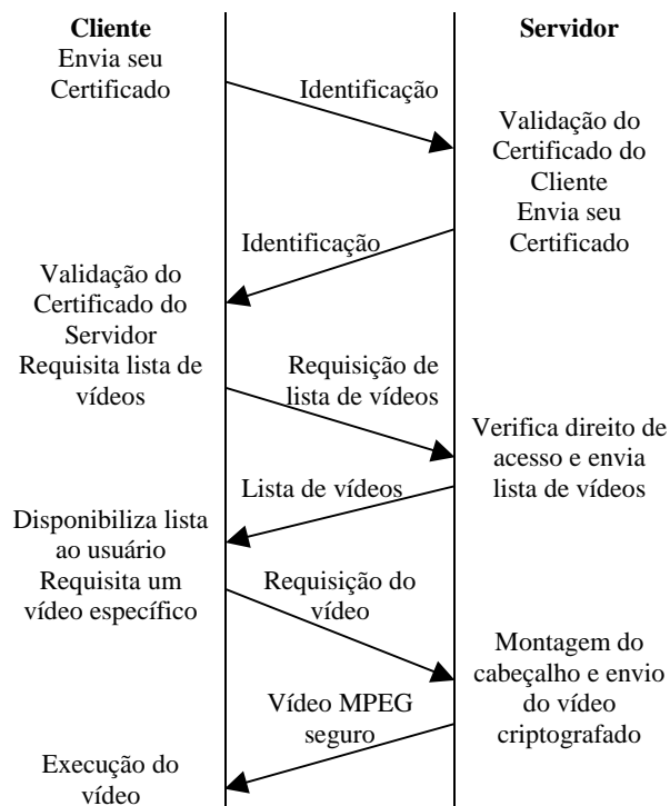
Figura 4: Diagrama de Tempo das Mensagens Trocadas entre o Cliente e o Servidor para Acesso ao Vídeo MPEG Seguro
