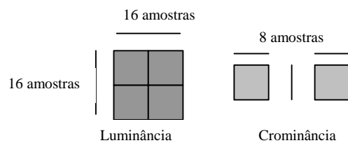
Figura 1: Constituição do Macrobloco MPEG
